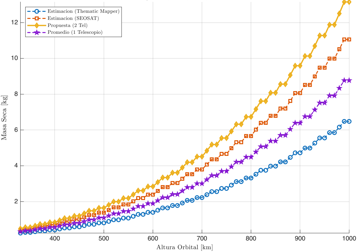
Comparativa de Masa Seca vs. Altura Config: 1 Sat, 2 Tel, Det 3, Refractivo
